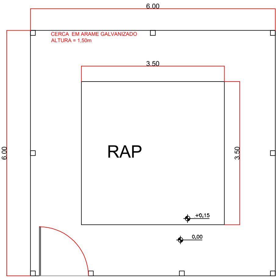
PLANTA BAIXA ESCALA 1-25 AREA: 36m 2
