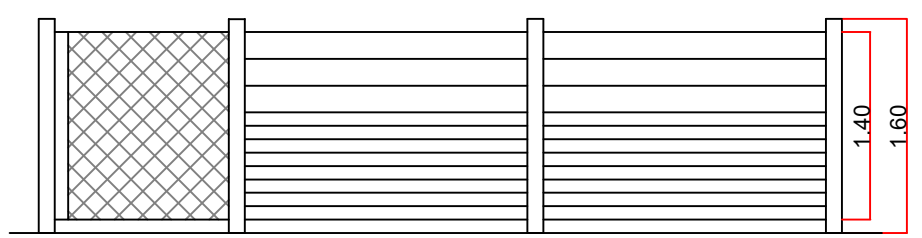
DETALHE CERCA ESCALA 1-25 CERCA EM ARAME GALVANIZADO
