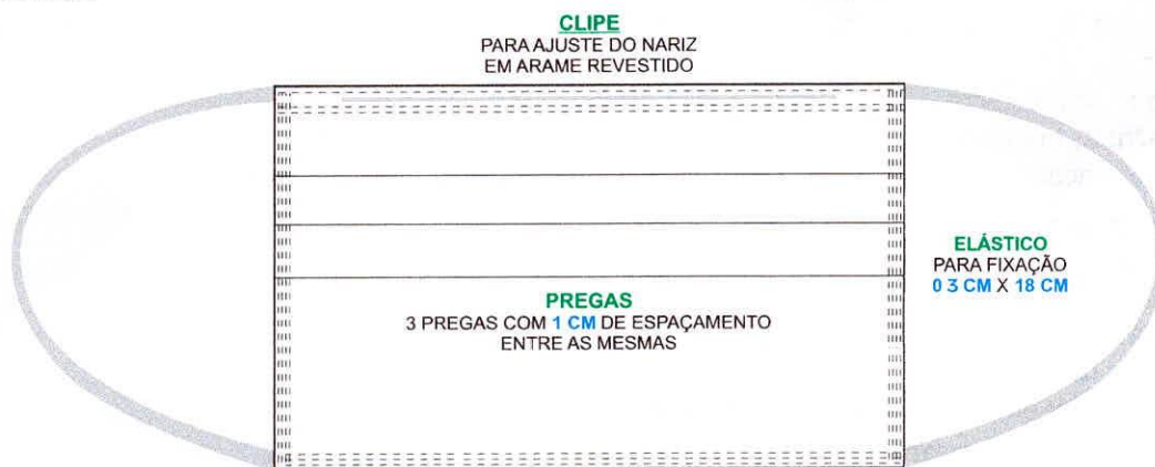
DESENHO TÉCNICO
