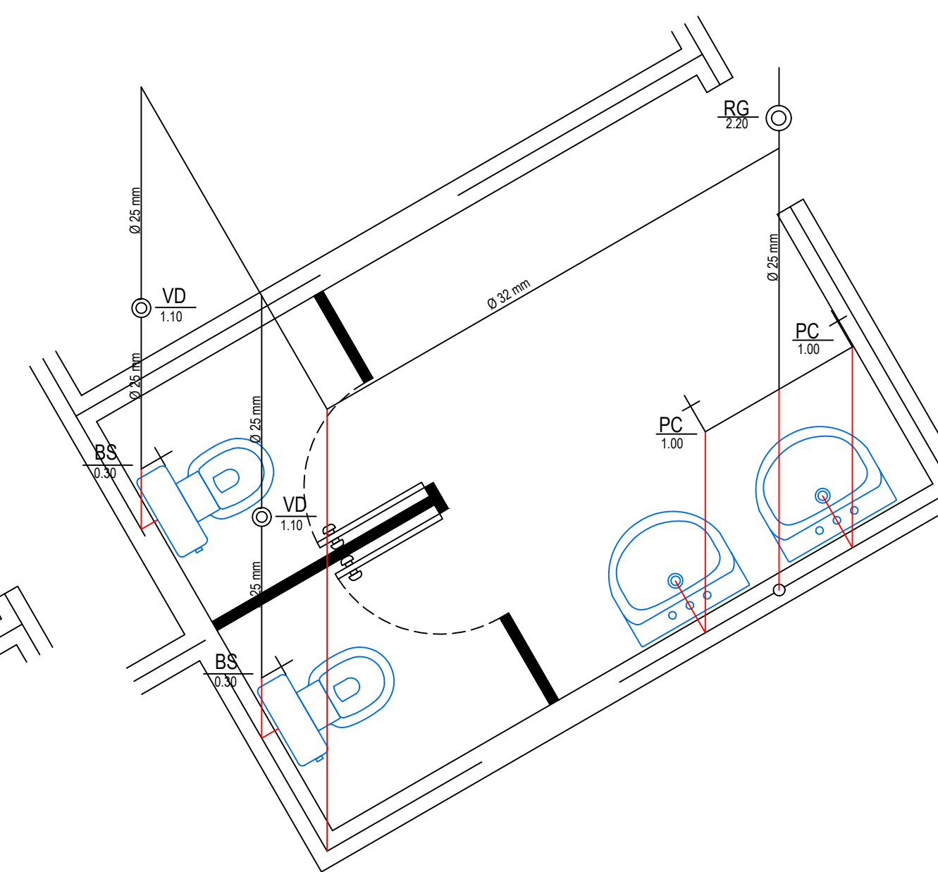
ISOMETRICO 03 ESCALA 1:25
