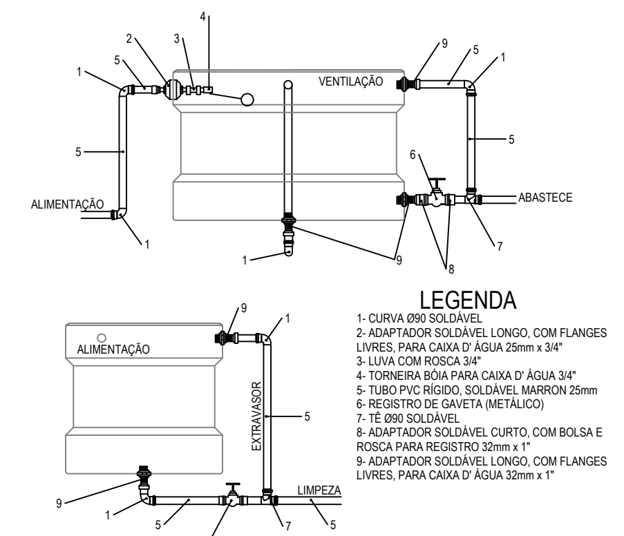
DETALHE - CAIXA D'ÁGUA 1.000 Lts SEM ESCALA
