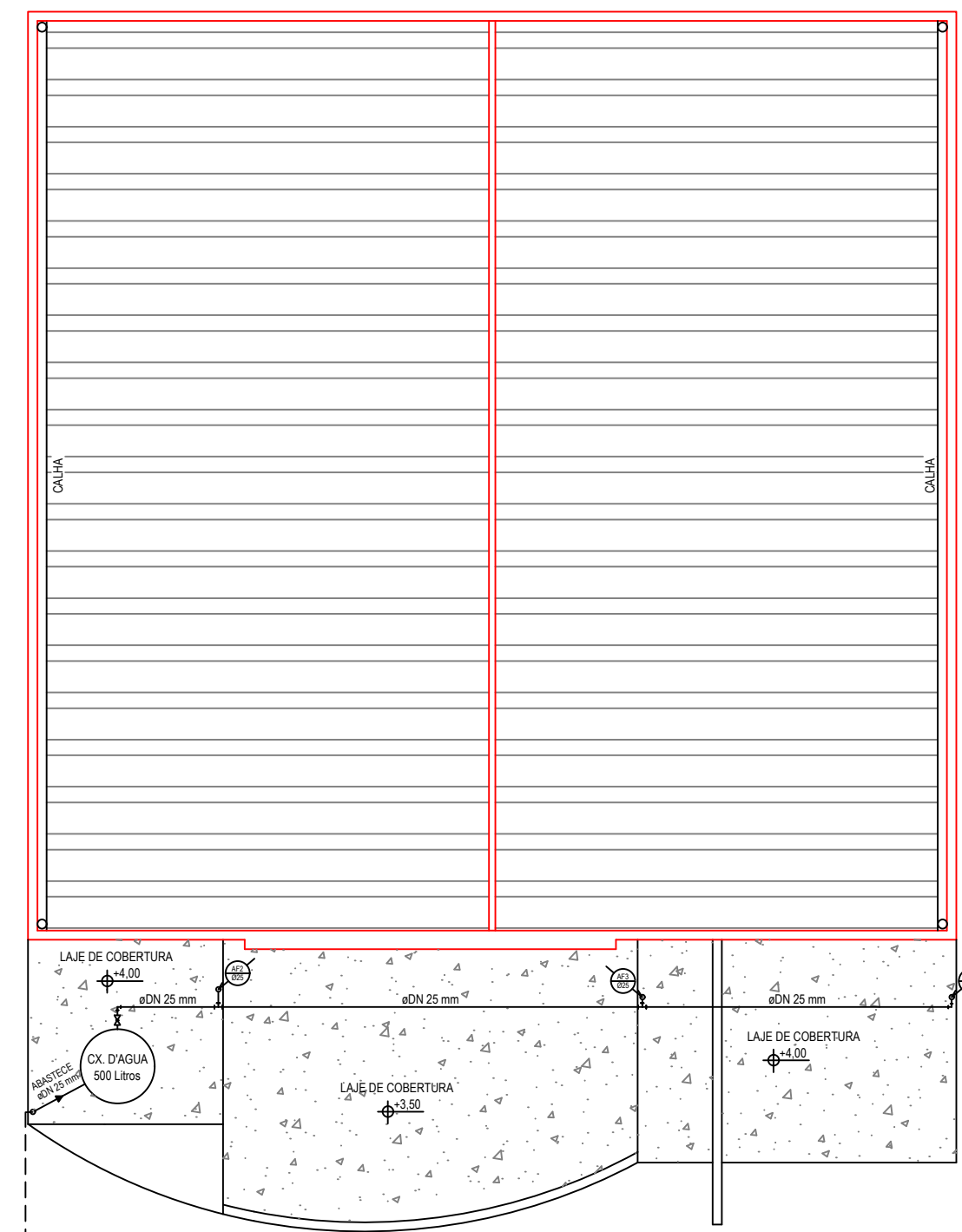
PLANTA DA COBERTURA
