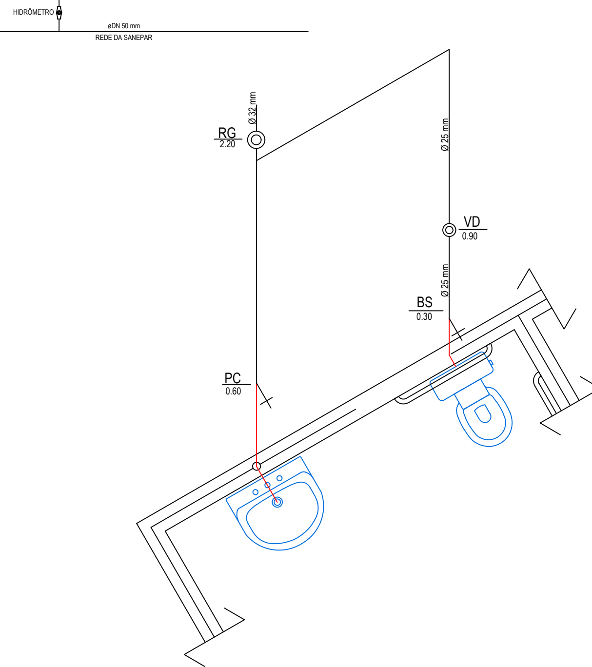
ISOMETRICO 01 ESCALA 1:25
