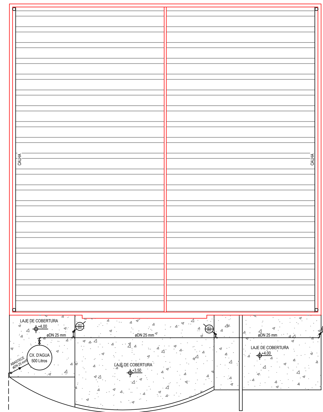
PLANTA DA COBERTURA HIDRÁULICA ESCALA- 1:100 OBS: A CX D'ÁGUA DERA APOIADA SOBRE A LAJE DA COBERTURA COM ALTURA DE 4M
