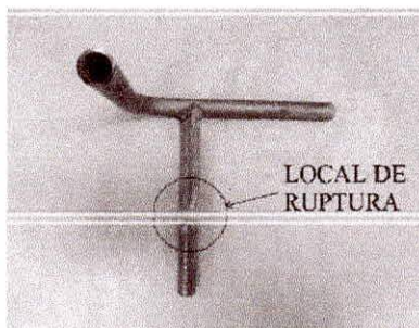
Foto 04 - Após o ensaio
