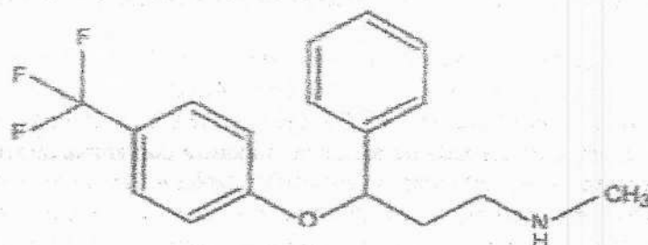
Figura 1 - Estrutura química da Fluoxetina
