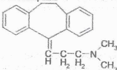
Figura 2 - Fórmula estrutural da amitriptilina
