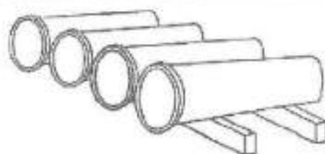
Figura G.1 — Apoio dos tubos ponta e bolsa quando estocados na horizontal
