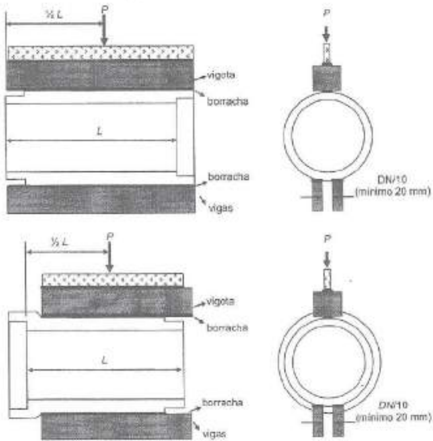
Figura F.1 — Esquema do ensaio para tubo ponta e bolsa e macho e fêmea
