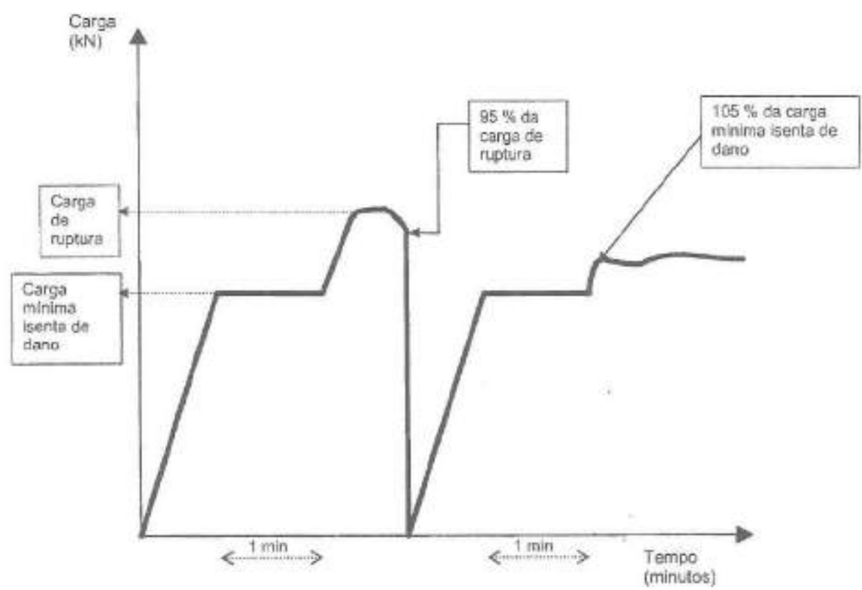
Figura F.2 — Esquema do plano de carregamento do ensaio
